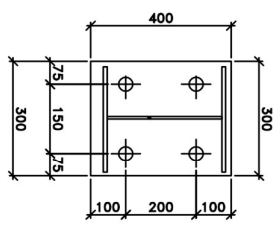
BASE PLATE D2
